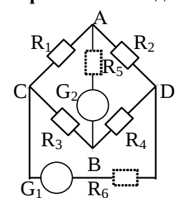
Рис.2.2.Схема моста
