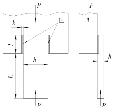
Рис. 1. Фланговый сварной шов. Сжатие.
