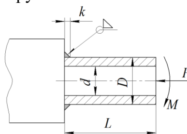
Рис. 4. Тавровое соединение. Кручение.
